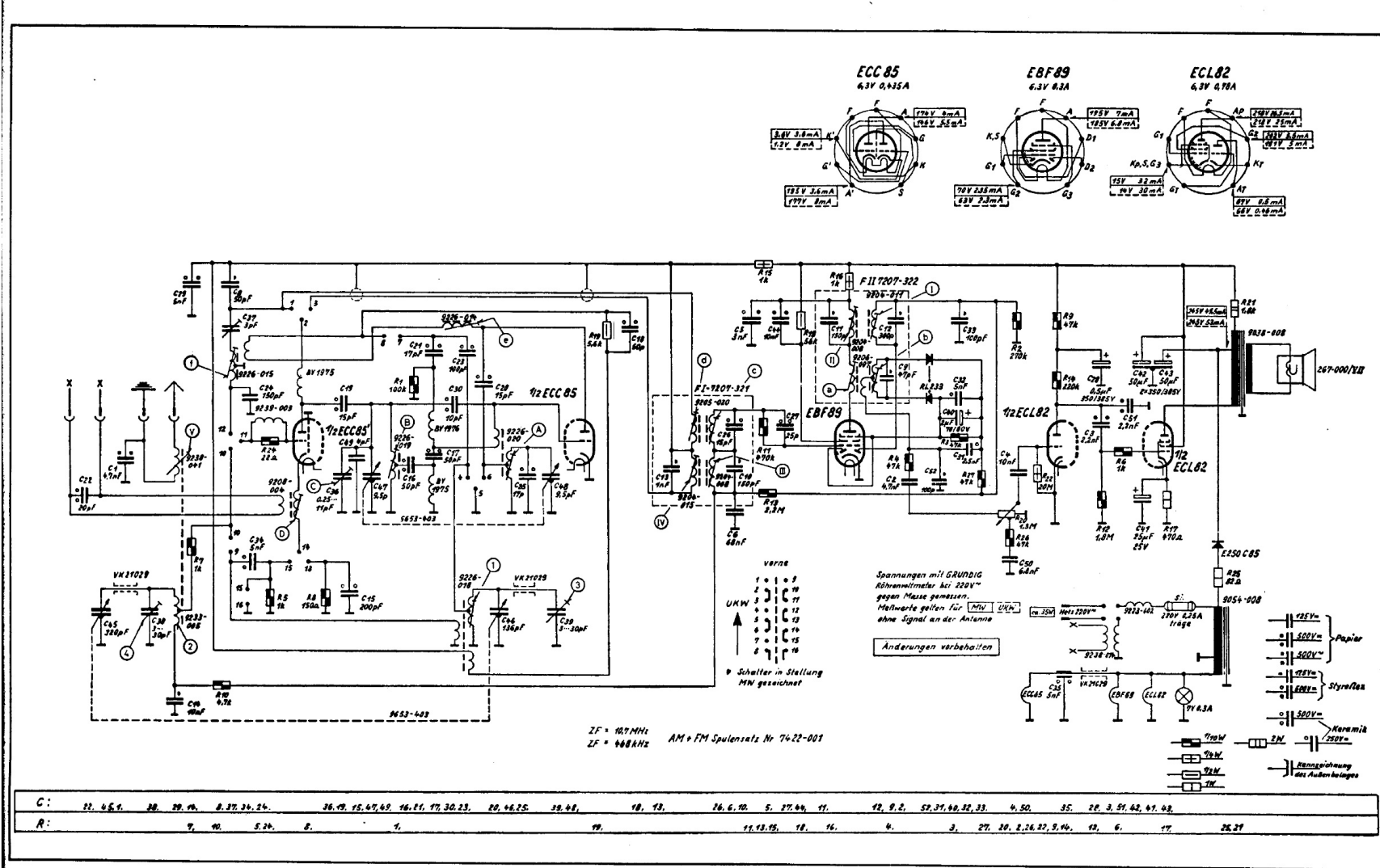
GRUNDIG (Radio Werke Fürth/Bay) - Mod. 85. Apparechio AM/FM a tre sole valvole, una coppia di cristalli di germanio per la rivelazione FM, e un rettificatore a selenio. Una gamma onde medie e una gamma onde ultracorte. Media frequenza AM a 468 kc/s e MF/FM a 10,7 Mc/s. Consumo CA 35 watt.
